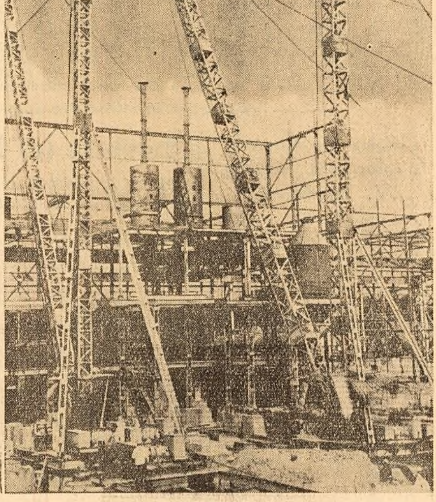
Construcția unei moderne fabrici de zahăr la Padokan (Indonezia).
