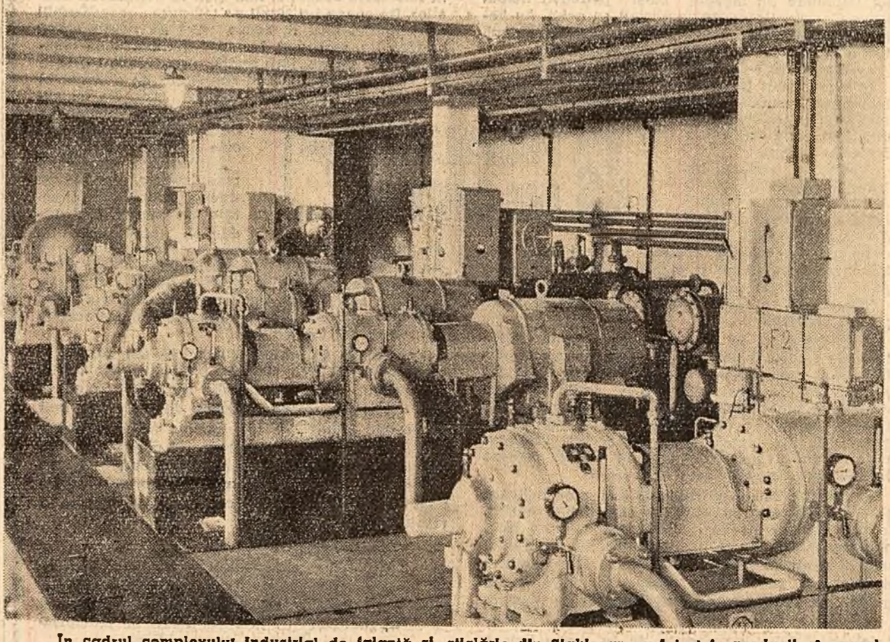
În cadrul complexului industrial de țelamă și sticlărie din Sighișoara a intrat în producție în acest an fabrica de sticlă de ambalaj. În fotografie: Aspect din sala compresoarelor.
