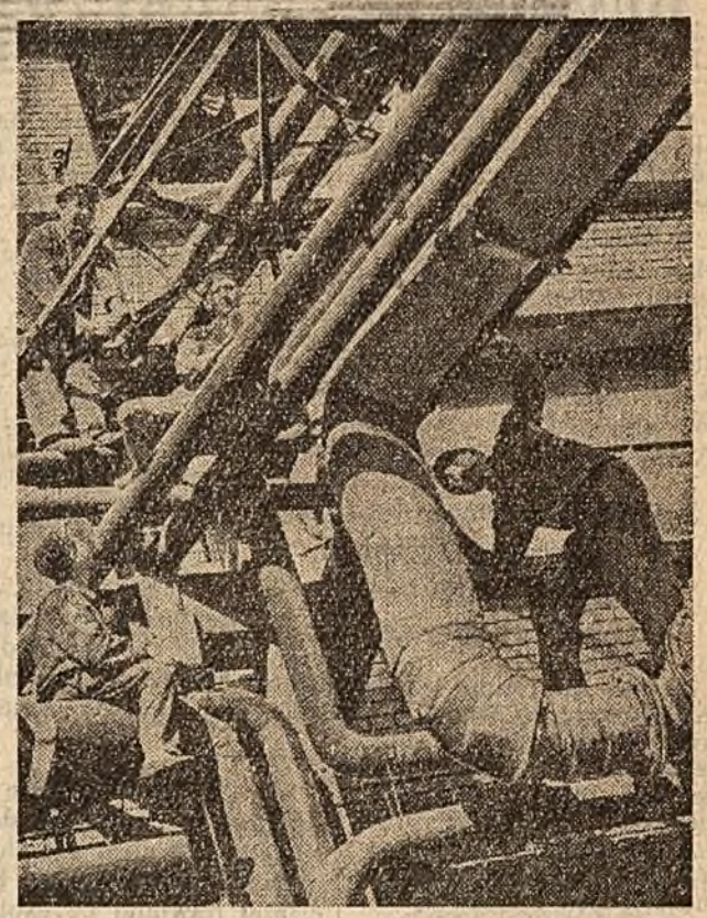
La uzinele „Grivița Roșie”-București, pregătirile pentru iarnă sînt avansate. Multe din măsurile prevăzute au și fost îndeplinite. În fotografie: Echipa de întreținere condusă de maestrul Ștefan Luntrașu lucrează la izolarea unor conducte cu aburi. (Foto: R. Costin)
