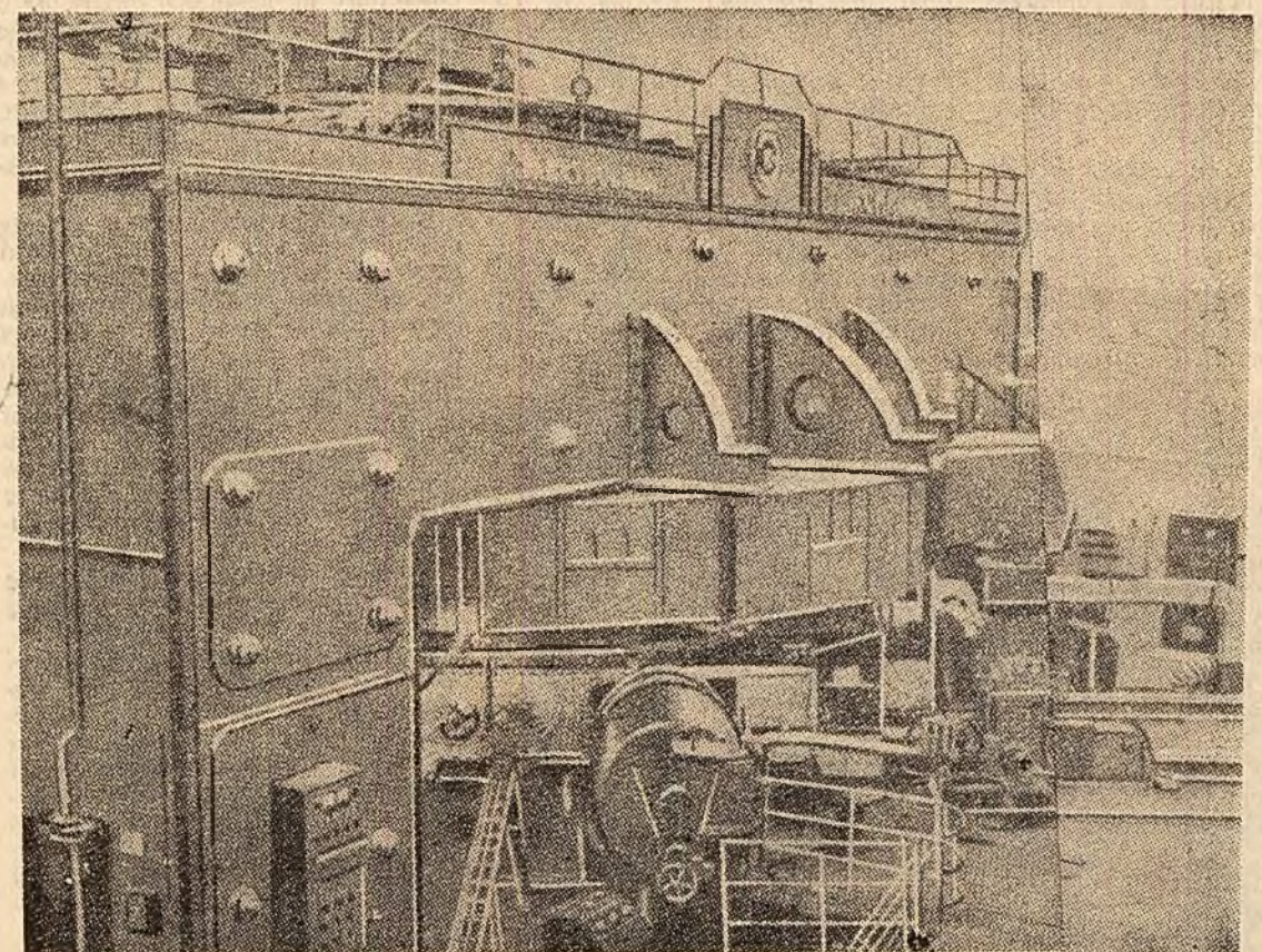
Sincrociclotronul de 680 milioane electronvolți, construit de oamenii de știință sovietici și instalat la Institutul unificat de cercetări nucleare de la Dubna, este un instrument pentru studiarea particulelor elementare.
