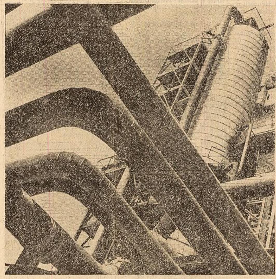
Coloanele rafinării (Aspectul nr. 10 — Onești).
