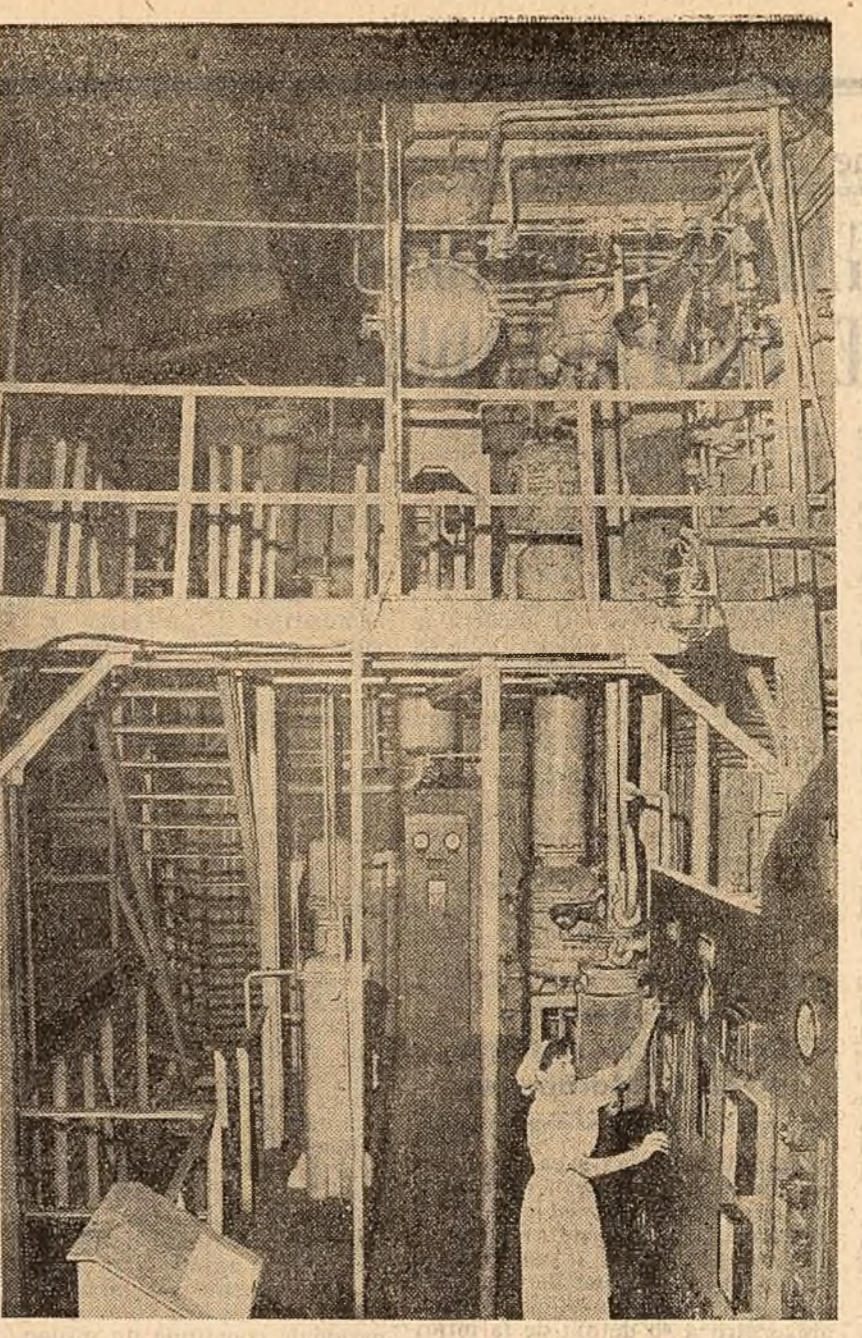
Instalația de distilare a monomerilor de la fabrica de produse chimice din Turda.
