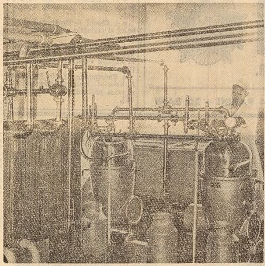
Fabrica de produse lactate de la Cisluru Seculesc. Aspect din secția de pasteurizare a laptei. (Foto: R. Costin)
