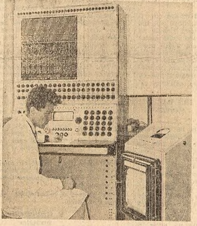
Mașina de calcul analitic pentru studiul reactorilor nucleari. În fotografie: Ing. Cornel Tapu, unul dintre realizatorii mașinii, urmîrindu-l funcționarea. (Foto: Agerpres)
