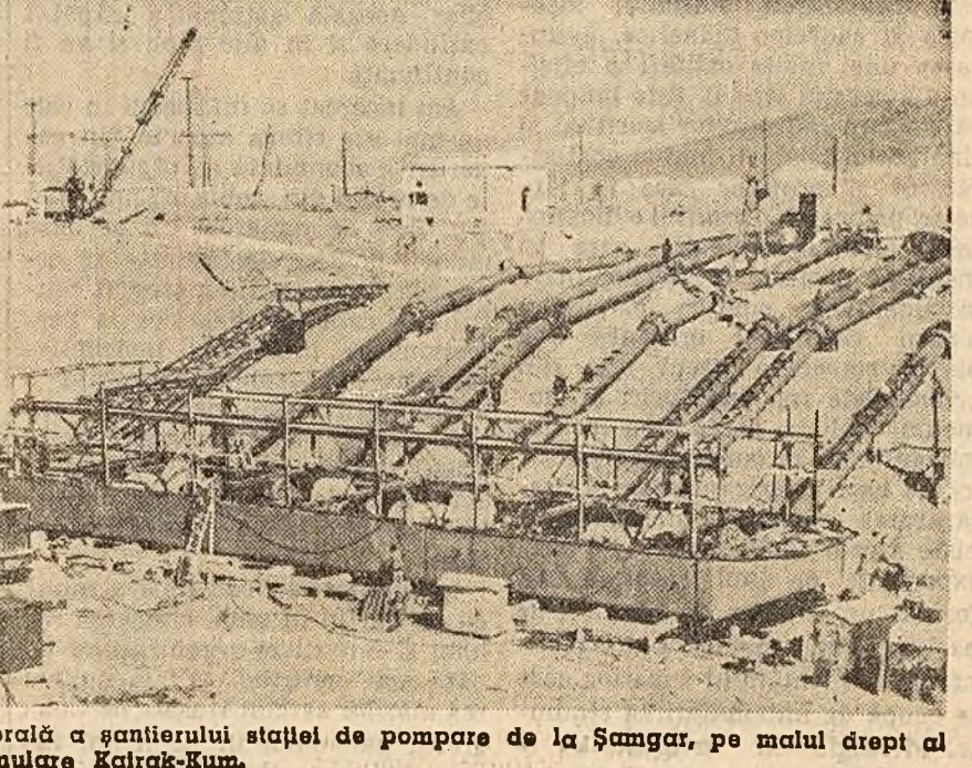
Vedere generală a șantierului stației de pompare de la Șamgar, pe malul drept al lacului de acumulare Kairak-Kum.
