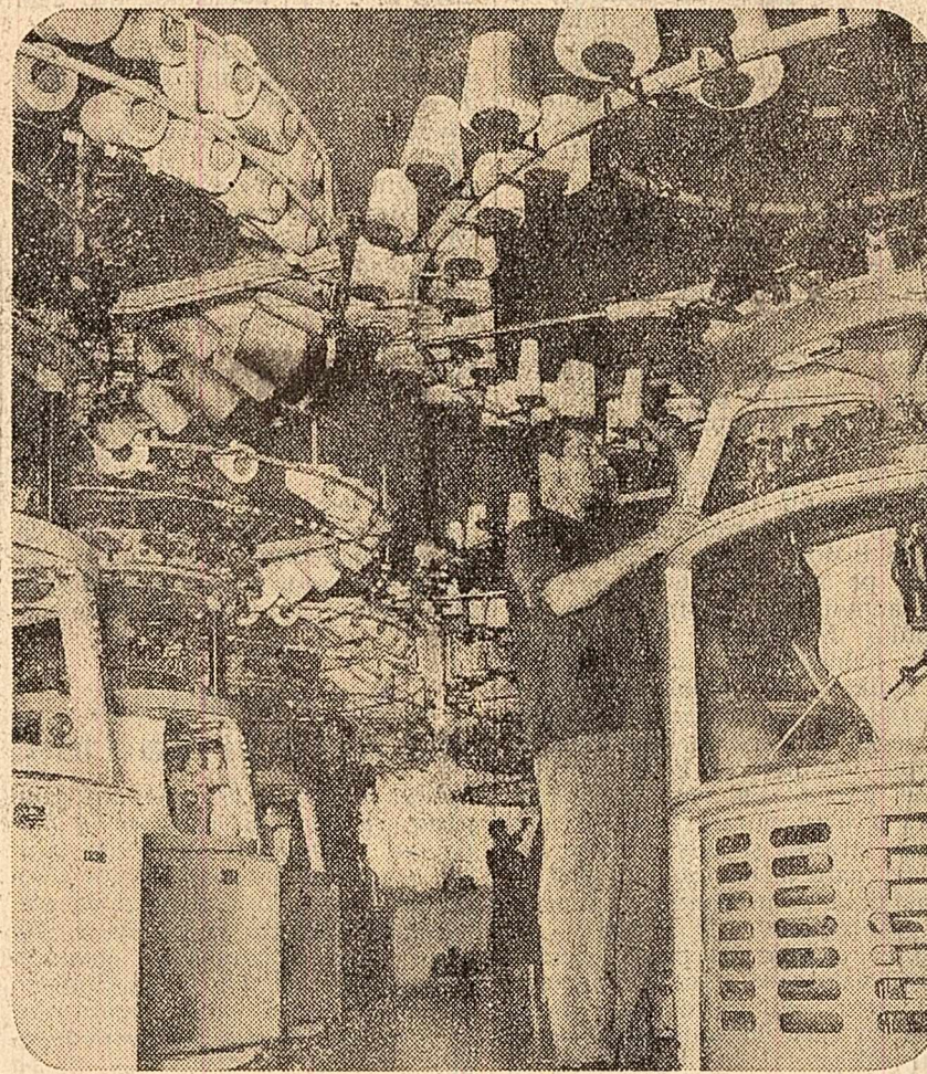
Fabrica de confecții și tricotaje din București. Aspect din secția de mașini circulare de tricelat. (Foto: Agerpres)
