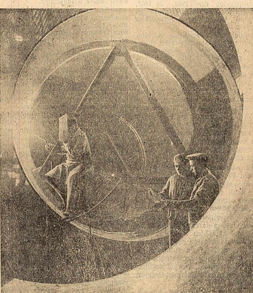
Căminii Emil Fintineru și Constantin Badaș de la Uzina de utaj chimic și petroler din Capitală, consiliul planul de asamblare a unui rezorvor înainte de sudarea cercurilor de încălzire. (Foto: Agerpres)
