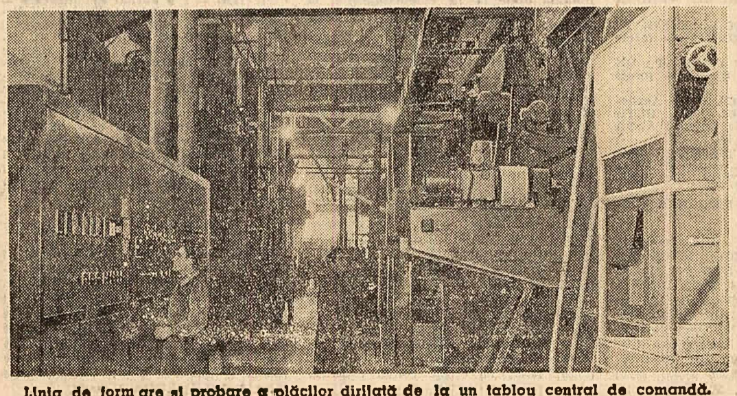
Linia de formare și probare a plăcilor dirijată de la un tablou central de comandă.
