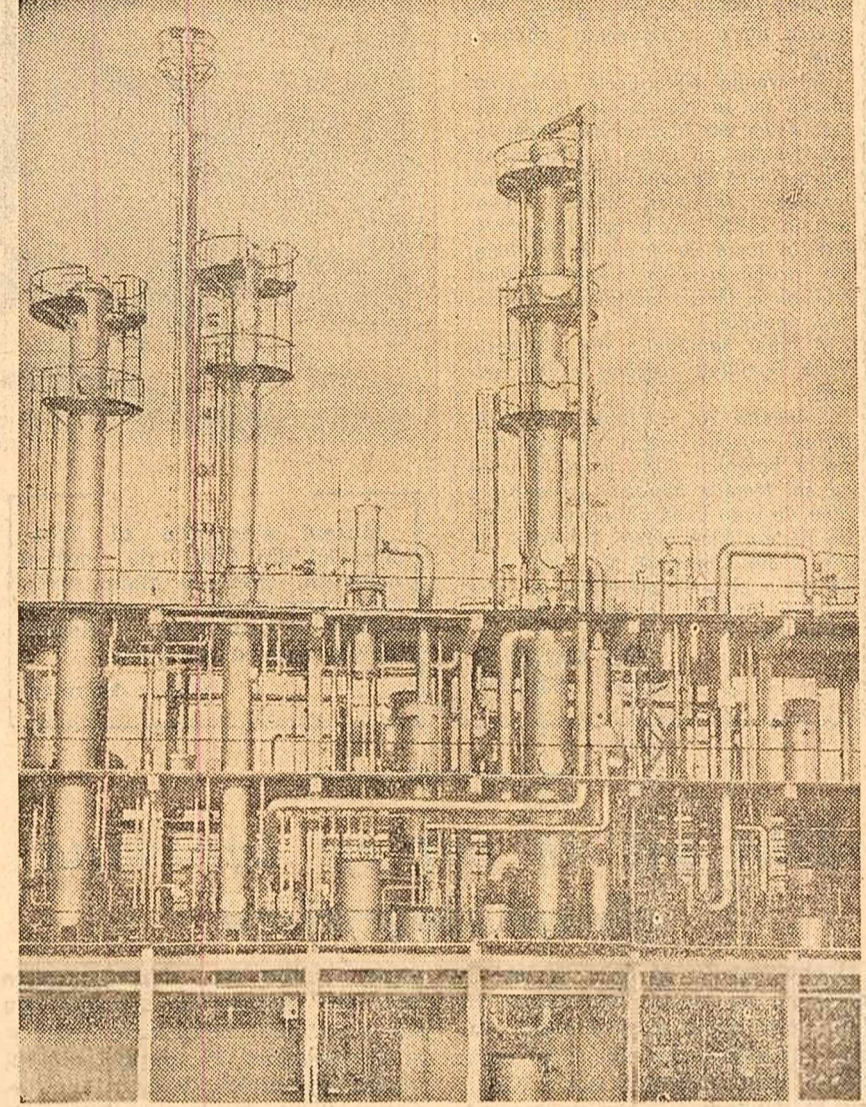
Instalația de acelență a uzinei de fibre sintetice Săvești. (Foto: Gh. Vințilă)
