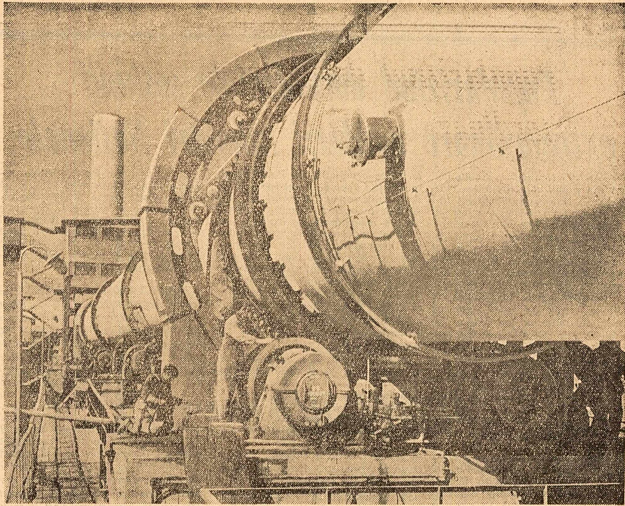
Noua linie tehnologică de 800 tone de klinker de la Fieni este una din cele mai mari și mai moderne linii de acest fel construite în țară. (Foto: R. Costin)
