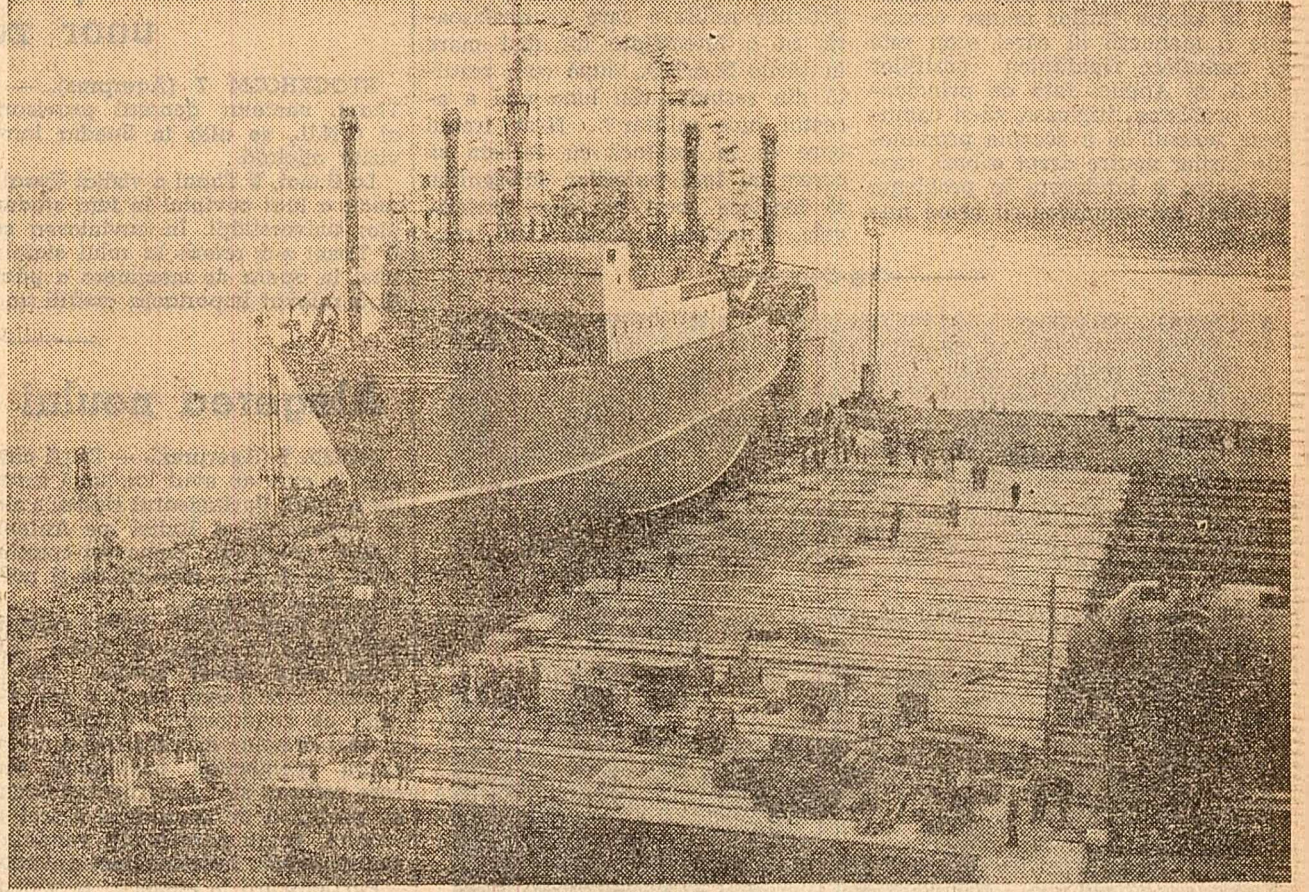
Recent, la șantierul naval din Stralsund (R.D.G.), a fost experimentată cu succes o instalație automată pentru ridicarea și lansarea la apă a vaselor. Ea a fost produsă de o întreprindere din Leipzig. Instalația poate ridica și lansa la apă vase cu o greutate proprie pînă la 3.000 de tone. În fotografie: lansarea la apă a unui vas de pescuit.
