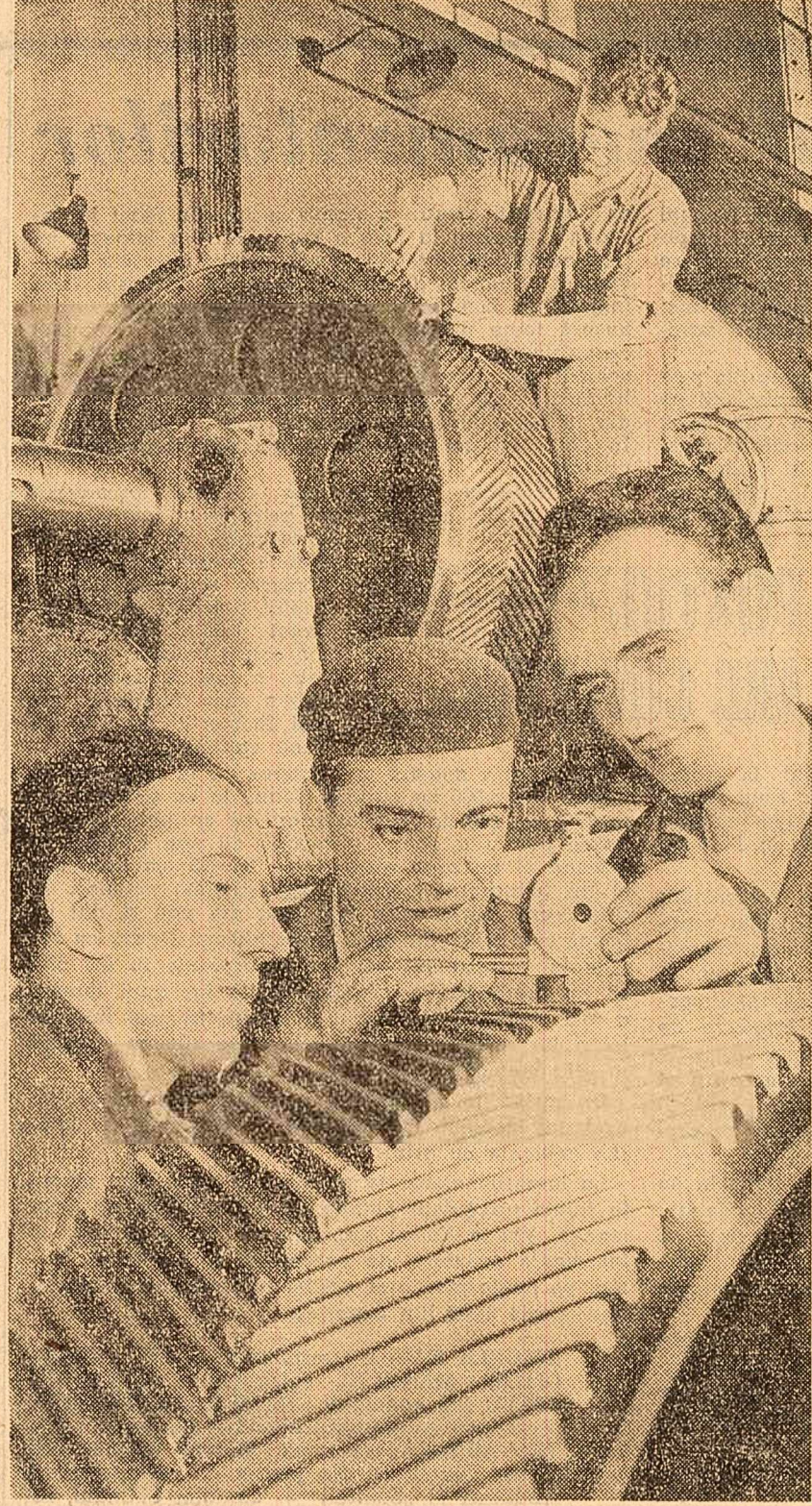
Uzinele de uzină chimică din București: Șandor Anton, frezor, Emil Varlam, recepționar, Ion Gheorghie, maistru, (în prim plan) făcînd o ultimă verificare a unei roți danturate lucrate în uzină.
