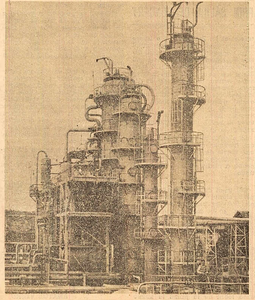
Rafinăria Onești — vedere parțială (Foto: Gh. Vințu)
