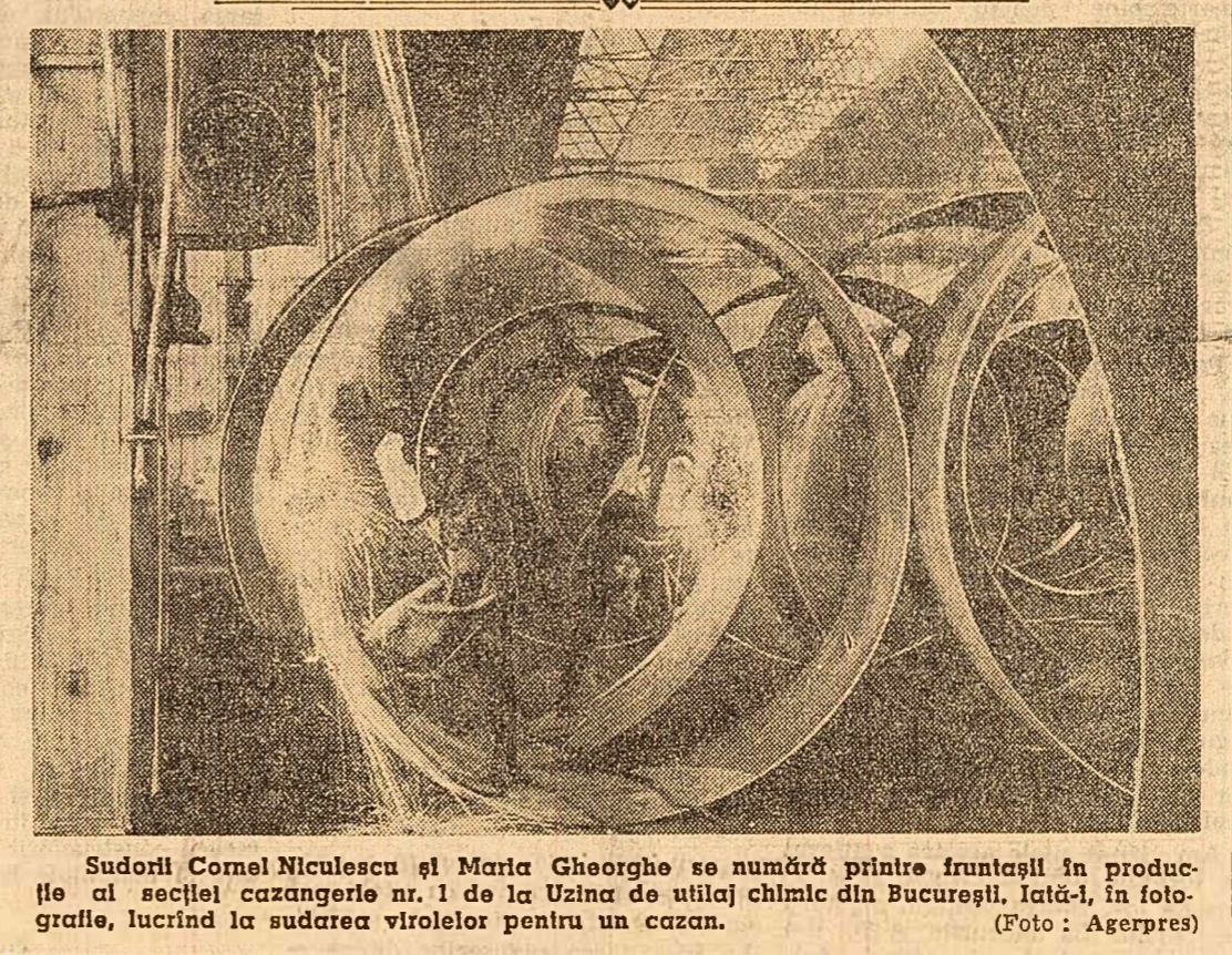
Sudorii Cornel Niculescu și Maria Gheorghe se numără printre frunțașii în producție al secției cazangerie nr. 1 de la Uzina de utilaj chimic din București. Iată-l, în fotografie, lucrînd la sudarea virolelor pentru un cazan.
