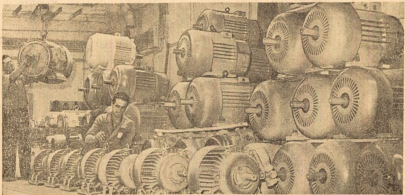
Colecția Uzinelor de mașini electrice din București a produs în acest an, peste plan, circa 300 mașini electrice și a realizat economii în valoare de 867.000 lei. În fotografie: Un nou lot de motoare electrice gata de expediție. (Foto: R. Costin)
