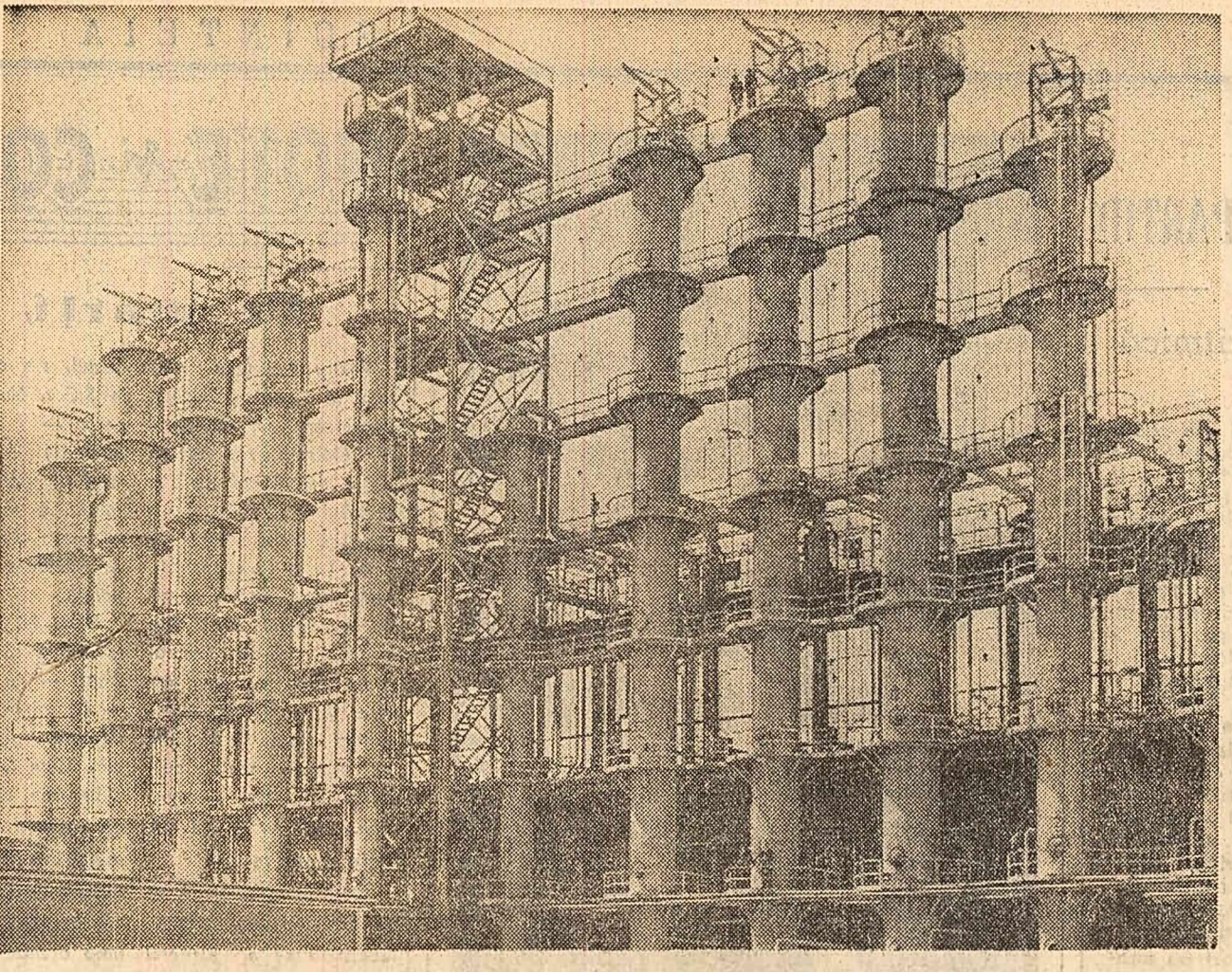
Instalația de obținere a izopropilbenzenului de la Combinatul de cauciuc sintetic și produse petrochimice Onești. (Foto: Gh. Vințilă)
