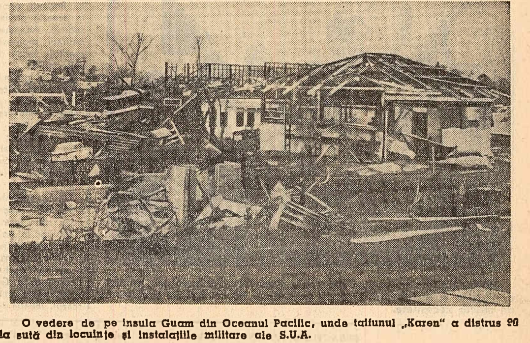
O vedere de pe insula Guam din Oceanul Pacific, unde tainful „Karen” a distrus 80 la sută din localitate și instalații militare ale S.U.A.
