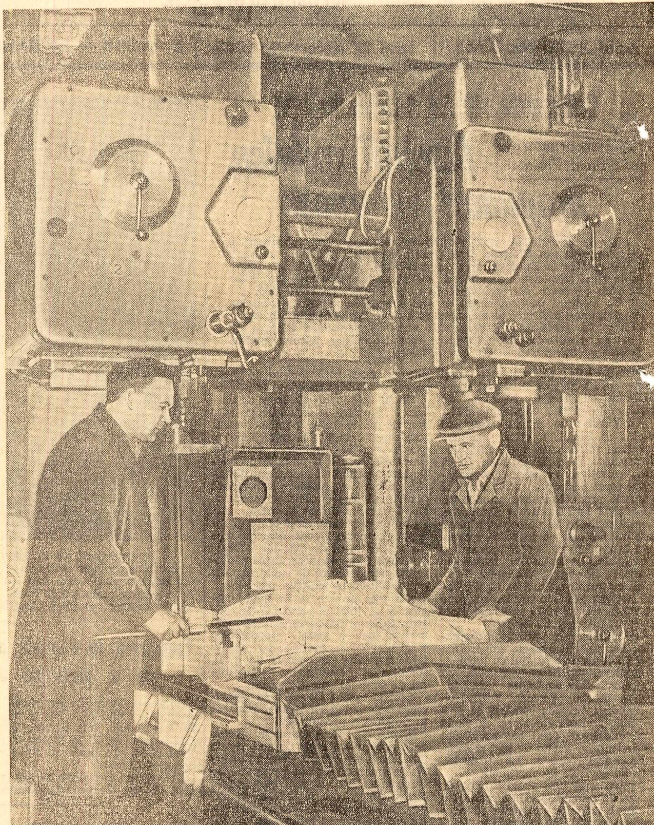
Mașina portată de frezat - utilaj modern cu care a fost înzestrată întreprinderea. La această mașină se produc bănușii și alte piese mari ale noilor produse.
