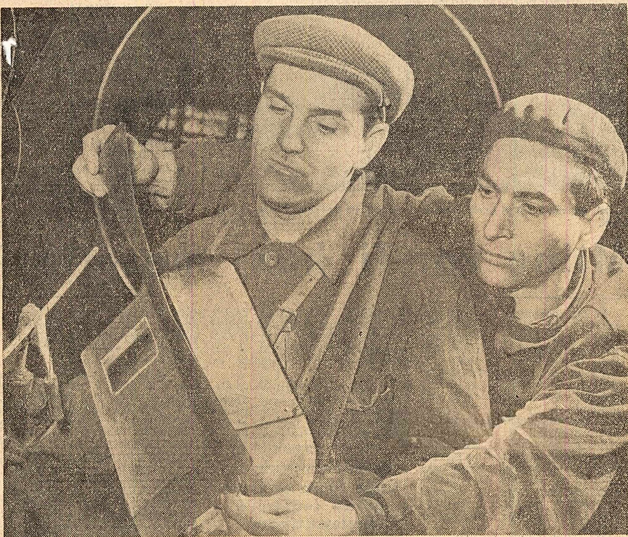
Craițuirea cu arc electric și aer comprimat este o nouă metodă care se aplică în sectorul cazangeriei al Uzinelor „23 August” din Capitală. Față de vechiul procedeu de craițuire cu aparatul pneumatic, prin folosirea acestei metode se obține o creștere de 50 la sută a productivității muncii, se elimină în mare măsură zgomotul din sector, îmbunătățindu-se astfel condițiile de lucru. În fotografie: Cazangii Alexandru Costescu și Nicolae Rădulescu stabilesc, pe baza indicațiilor controlului tehnic de calitate, porțuna cusăturii sudate unde vor aplica procedeu de craițuire „arc-aer”. (Foto: M. Andreescu)
