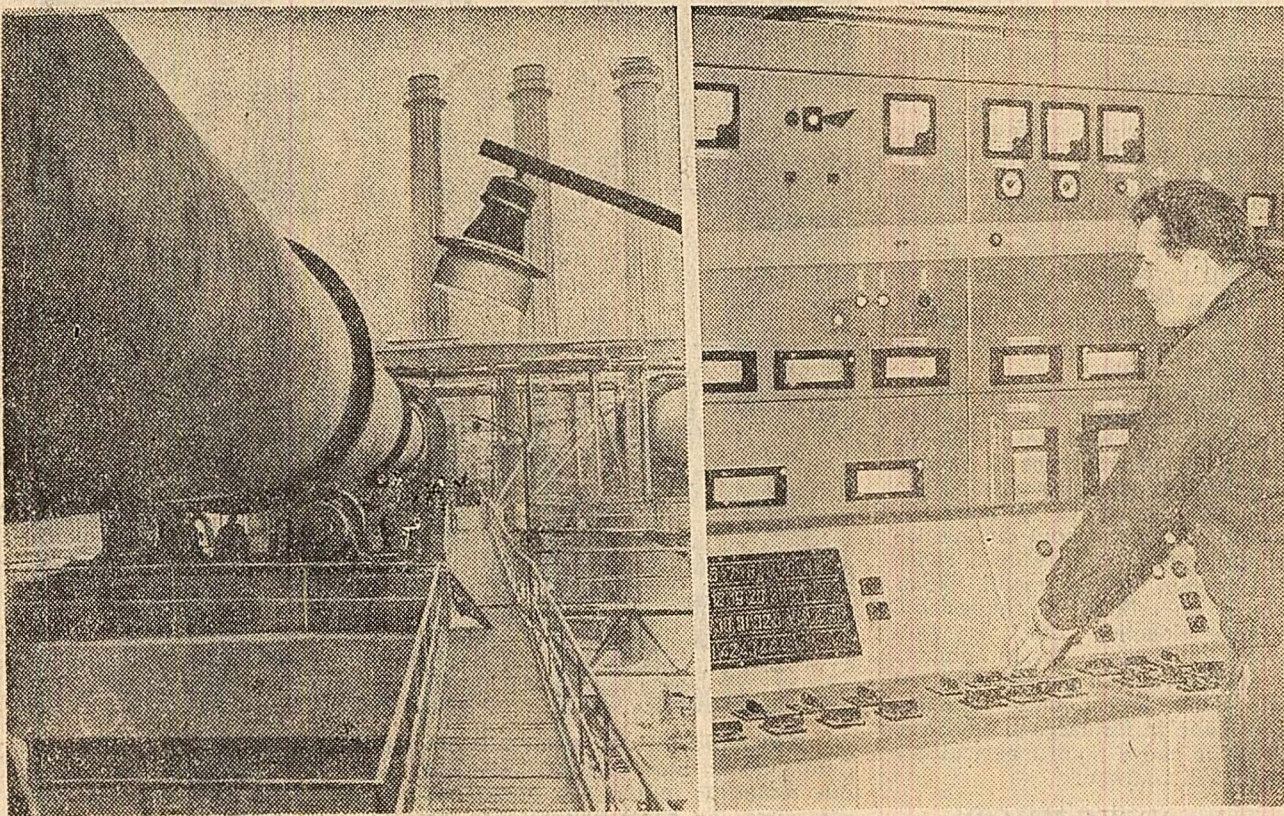
Fabrica de ciment „Victoria socialistă” din Turda. Cuprul de elincher cu o capacitate de 800 tone în 24 de ore (stînga); aspect din sala de comandă (dreapta). (Foto: R. Costin)
