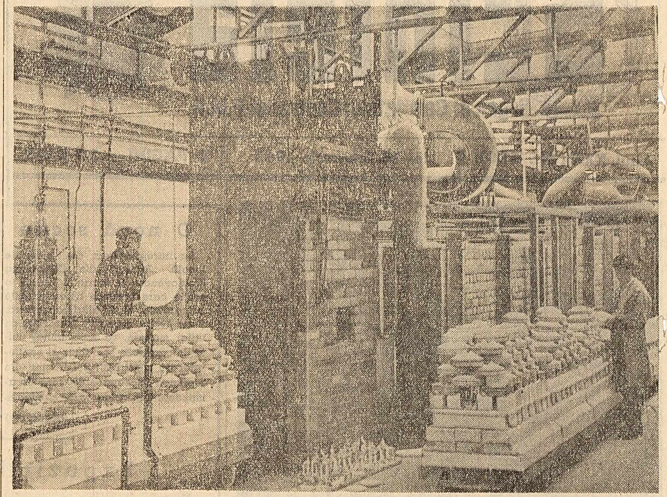
La întreprinderea „Petrolul”-Cluj. Aspect din sala cuptoarelor.
