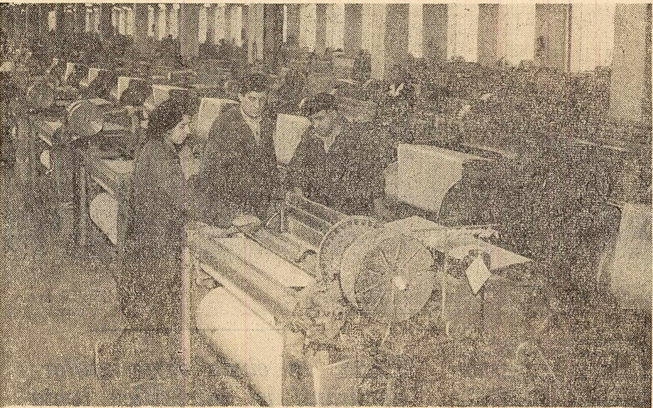
Doi din secțiile întreprinderii textile din Pitesti au fost de curând înzestrate cu războaie automate de țesut. În aceste secții productivitatea muncii și calitatea produselor a crescut simțitor. În fotografie: maistrul Traian Bădescu dând indicații tehnicilor George Ene și Maria Nedelcu asupra felului cum se lucrează la noile războaie automate de țesut.
