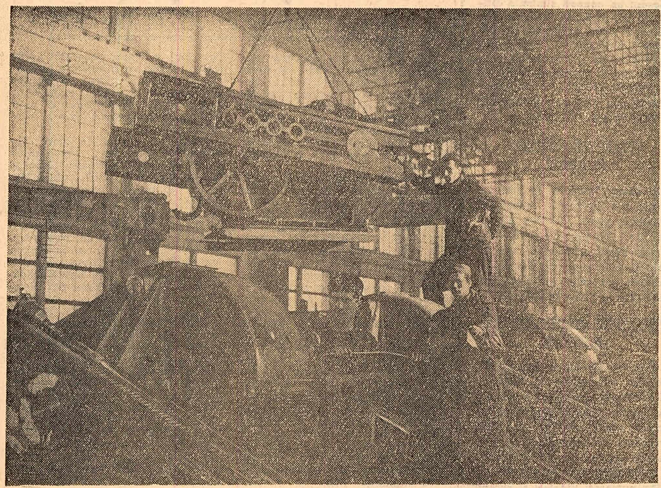
Aspect din sectorul de montaj-reductori al uzinelor „Vulcan” din Capitală. În fotografie: Șeful de schimb Viorel Gheorghe asamblînd, împreună cu cîțiva montori, reductori pentru industria petrolieră. (Foto: Agerpres)
