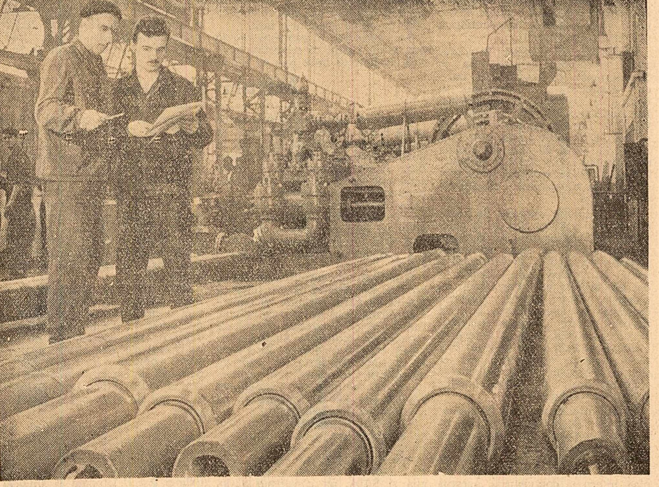
In secția montaj a Uzinelor „1 Mai”-Pliești se fac ultimele lucrări la un lot de turbine de foraj înainte de a fi expediate.
