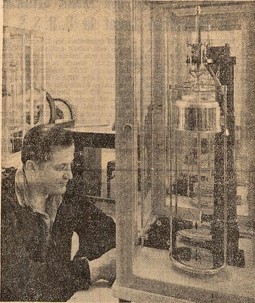
Metrologul Ioan Ardeleanu de la fabrica „Balanta” din Sibiu verifică o balanță etalon.
