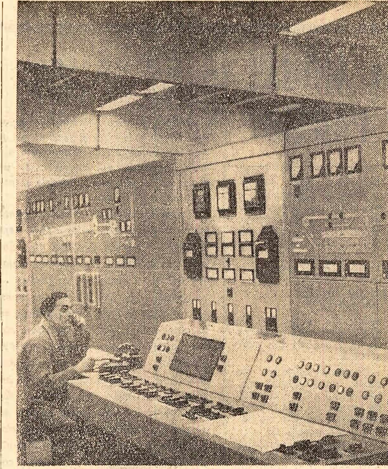
Fabrica de ciment „Victoria socialistă” din Turda. Se văd cele trei cupatoare de clincher, intrate de curînd în funcțiune. De la tabloul de comandă, muncitorul Nicolae Ciocîrlan supraveghează desfășurarea procesului de producție.
