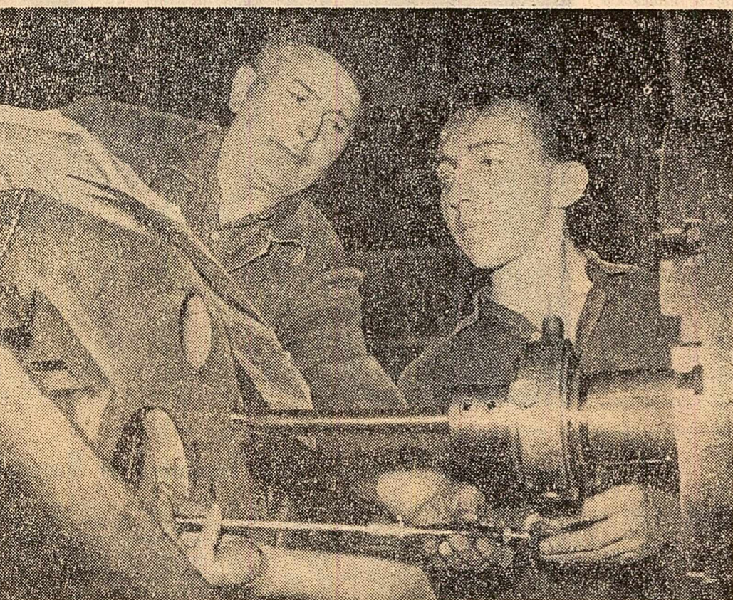
Strungarul Katanics Iosif dă indicații tîndrului Rusalin Lența la prelucrarea suportului de la agregatul pentru așchierea carterului motorului locomotivei Diesel electrice. Acest utilaj modern, proiectat de biroul tehnologic al grupului tehnic L.D.E., contribuie la mărirea productivității muncii la operațiile de găurire și așchiere.
