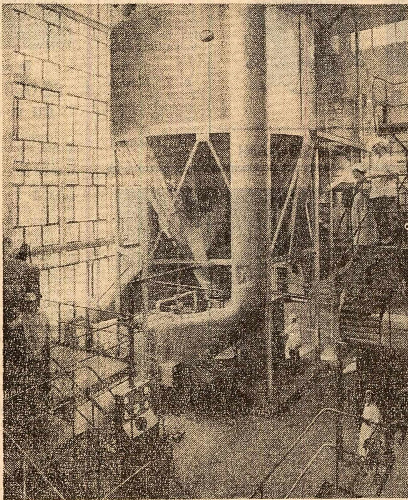
Instantanee de la fabrica de lapte „Barăul” din Cîmpulung Moldovenesc. În fotografia: stînga — instalația de concentrare și uscare a laptelui; dreapta sus: secția de ambalare a laptelui praf; fotografia de jos: vedere generală a fabricii. (Foto: Gh. Vințila)
