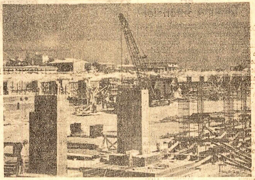
La vest de Havana, în provincia Pinar del Rio, se construiește cea mai mare centrală termoelectrică din Republica Cuba. Ea va intra în funcțiune anul viitor și va furniza energie electrică pentru Capitală și întreprinderile din două provincii. În fotografie: Un aspect de pe santierul centralei termoelectrice.
