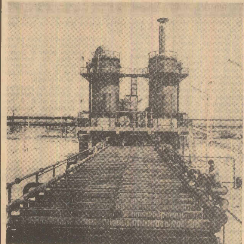
La Tarnobrzeg, în R. P. Polonă, au fost descoperite însemnate zăcăminte de sulf. Aici s-a construit un combinat pentru prelucrarea sulfului. În fotografie se văd, în prim plan, instalațiile de răcire.
