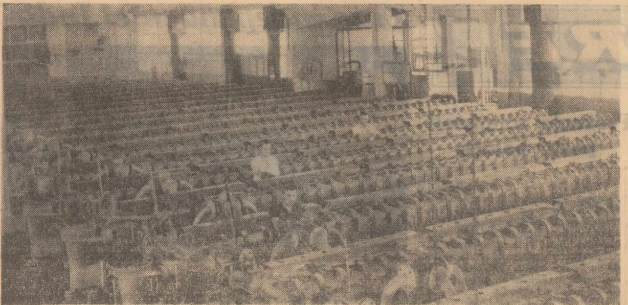
Instalația de electroliză a clorului de sodiu de la Uzinele chimice Turda. Operatorii Ștefan Șbirici, Olimpiu Hirț și Emil Băluțiu supraveghează celulele de electroliză. (Foto: Agerpres)
