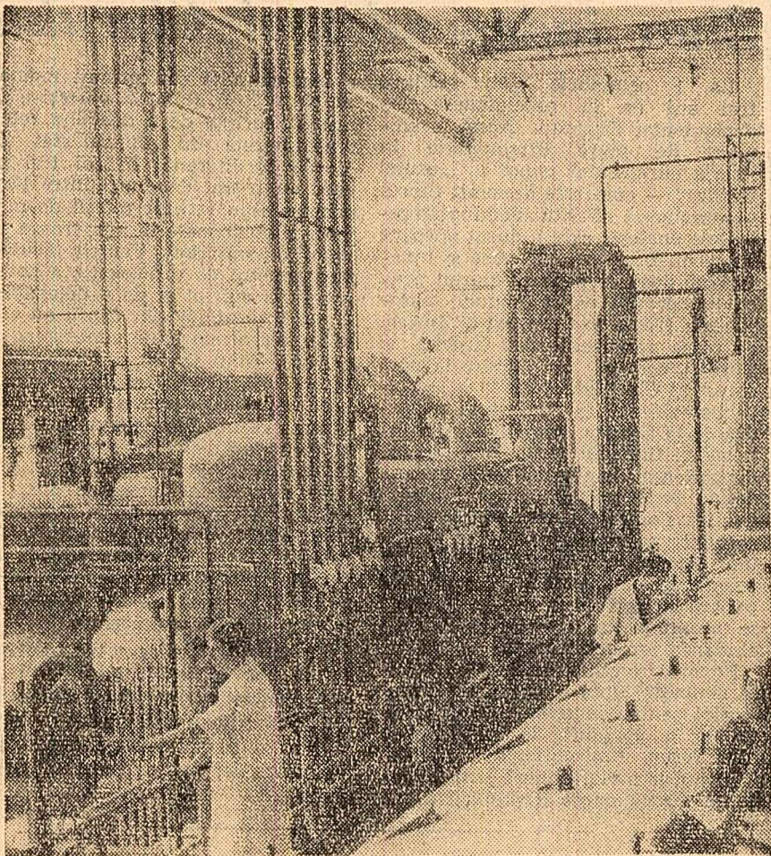
La fabrica „Unirea” Iași a început fabricarea uleiului comestibil din noua re- coltă de floarea-soarelui. În fotografie: Operatorii Vasile Pelu și Teodor Gherman ur- mănd funcționarea instalației de extragere a uleiului.
