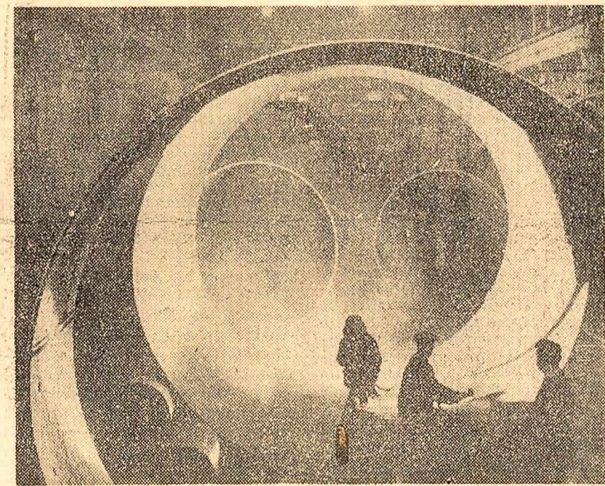
La cazangeria Uzinelor „Vulcan” din Capitală se aplică larg sudura automată, în special la construcția vicioare și recipientilor. Față de obiectivele proiectate de sudură, productivitatea muncii a crescut de aproape 6 ori. În 10 luni s-au realizat 90 000 metri liniari de sudură automată. O vicioară care se suda manual în 64 de ore, în prezent, folosindu-se sudura în mediu de bioxid de carbon, operația de asamblare s-a redus la numai 16 ore. Colectivul sectorului de cazangerie a realizat totodată, în 10 luni, economia în valoare de 2 600 000 lei. În fotografie: În cazangeria uzinei. (Foto: M. ANDRESCU)
