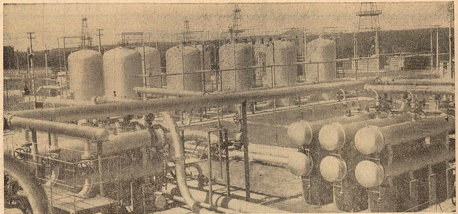
Din noul peisaj industrial al Olteniei: instalația de captare și dezbenzinare a gazelor de la Țicleni.
