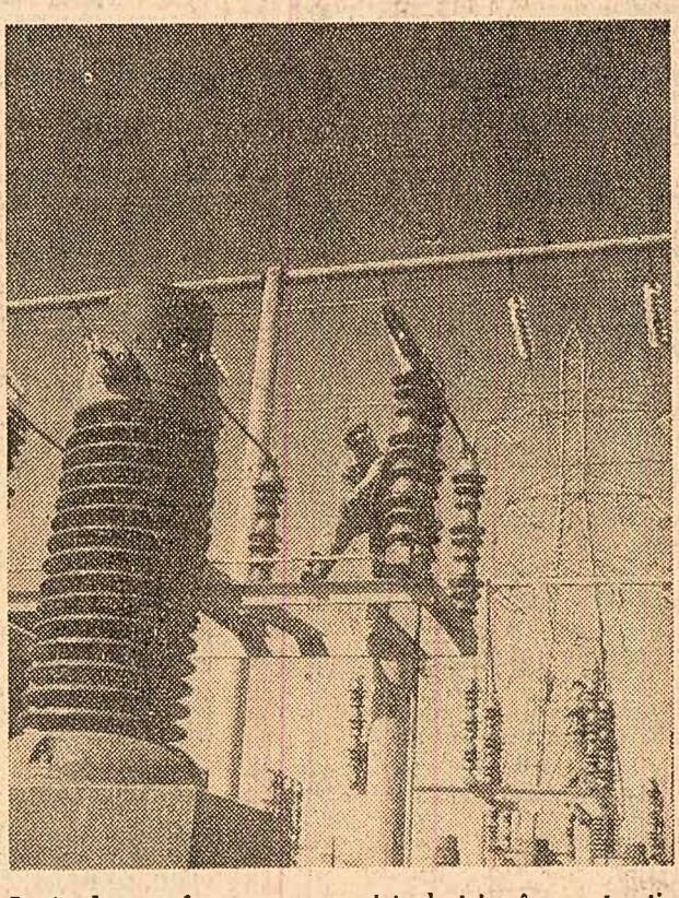
Stație de transformare a energiei electrice în construcție.
