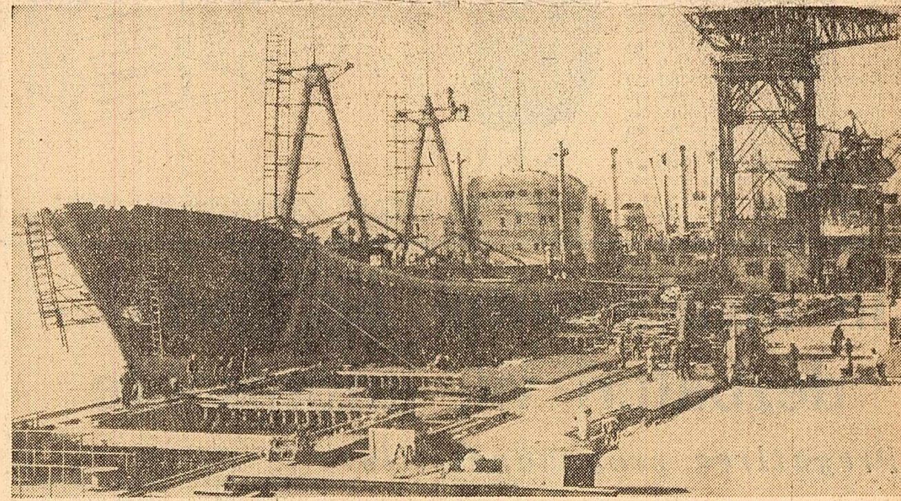
Cheul de armare a cargonților de 4.500 tone de la Șantierul naval Galați
