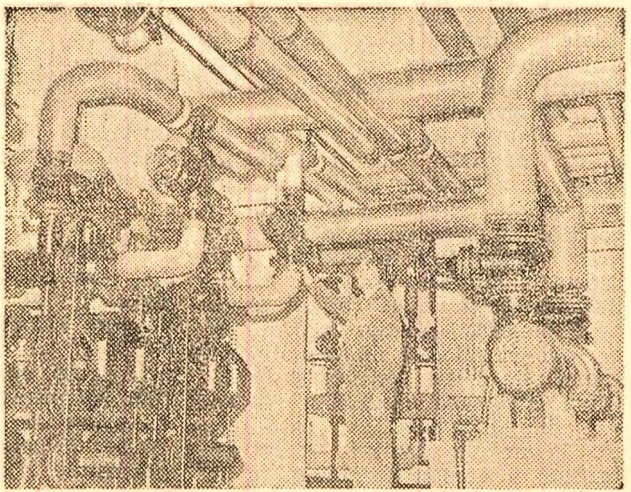
Punctul de termoficare de pe Calea Griviței nr. 164 din Capitală.
