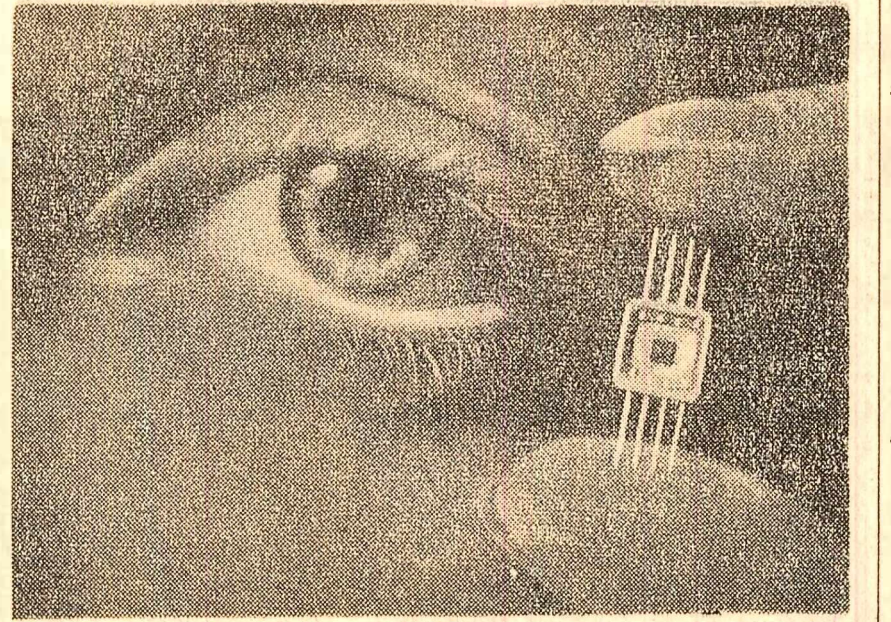
Miniaturizarea aparaturii este linia de dezvoltare a radiotehnicii moderne. Micul pătrat negru din fotografie, ceva mai mare decît un unghi chibrit, poate înlocui un aparat electronic alcătuit din 50 de tranzistori, diode, rezistențe și condensatori.
