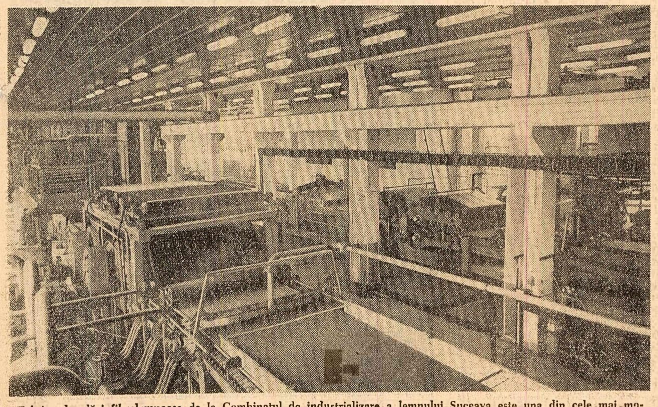
Fabrica de plăci fibrolemnoase de la Combinatul de industrializare a lemnului Suceava este una din cele mai moderne din țară. În fotografie: noile linii tehnologice ale fabricii.
