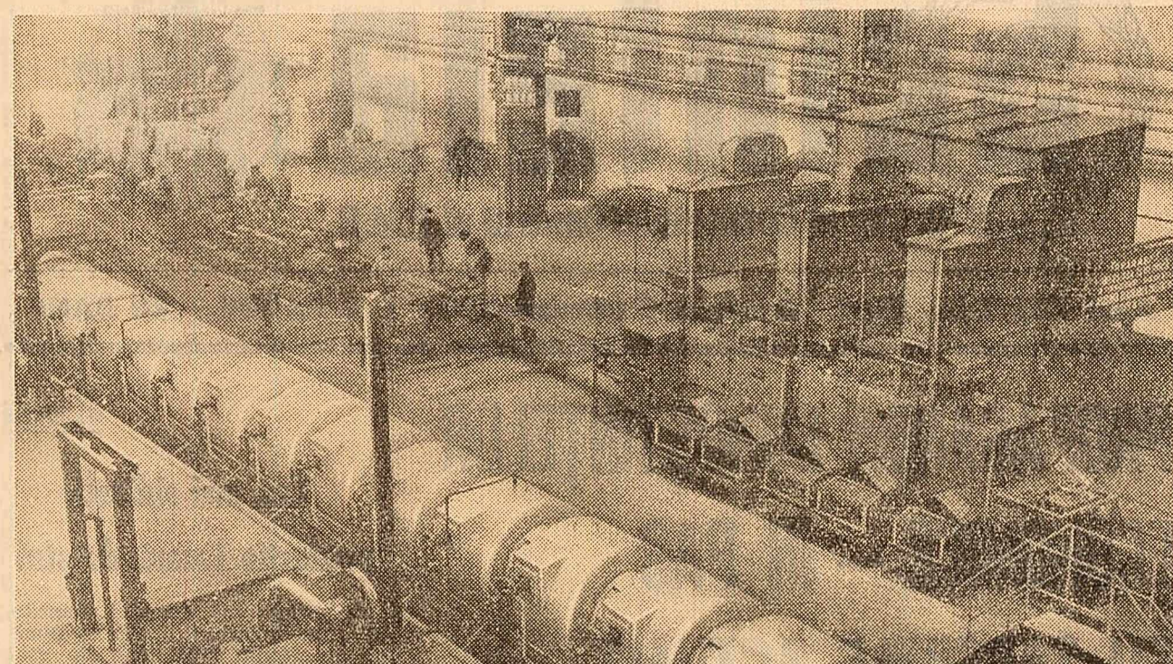
Uzina metalurgică din Iași. Liniă tehnologică de sudat țevi cu diametre de pînă la 4 joll.
