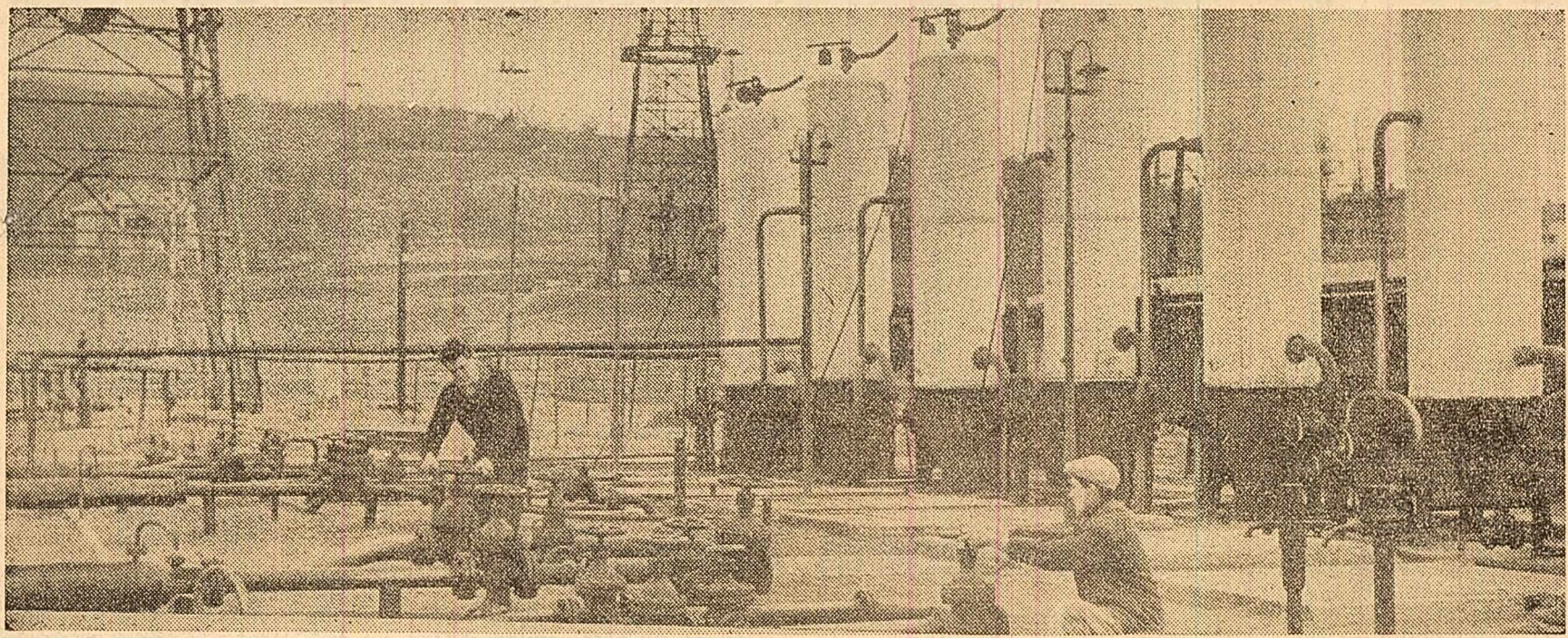
Schola Boldești, parcul de separatoare 700. Aici are loc separarea fiștelui de gaze. În fotografie: Operatorul Nicolae Bădescu, șeful parcului, împreună cu pompagii Nicolae Dobrescu execută extragerea dispozitivului de curățire a parafinei de pe conducte.
