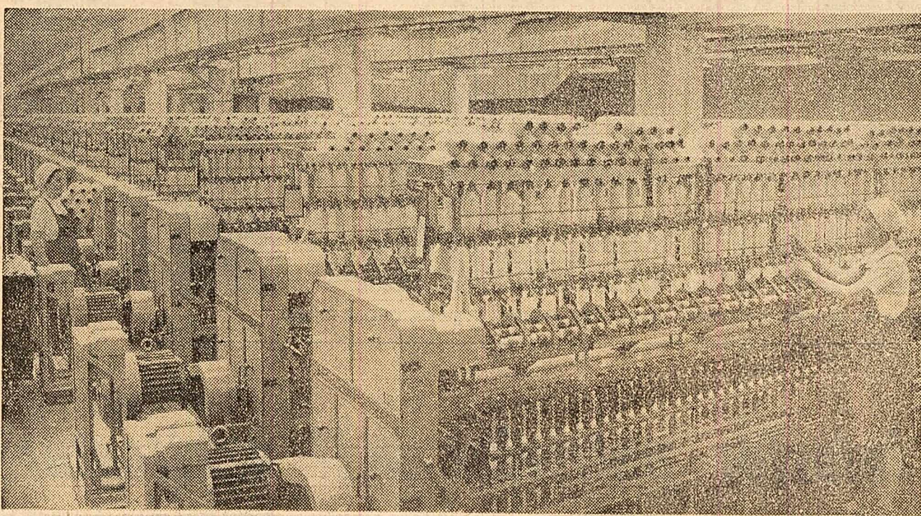
Hala de ringuri de la Filatura Românească de Bumbac-București
