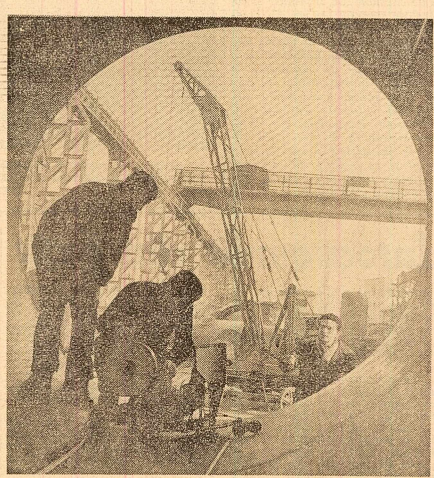
Uzina de ulei chimic din Capitală. Se execută o cusătură circulară la un recipient cu ajutorul aparatului de sudură automată.
