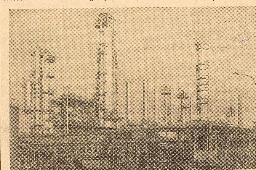
Instalații la rafinăria Schwechat
