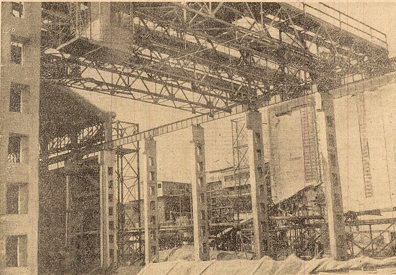
Pe șantierul Combinatului de îngrășăminte chimice din Turnu Măgurele, lucrările avansează în ritm susținut. Constructorii și montorii acordă o mare atenție respectării graficelor de execuție. În fotografie: Aspect de la depozitul de prăjit, unde se fac în prezent ultimele lucrări de finisaj.
