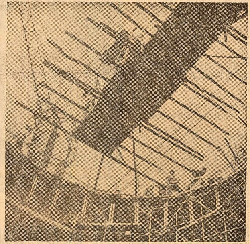
Turnarea betonului în cofraje gîslante la turnurile de granulare. Foto: R. Costin
