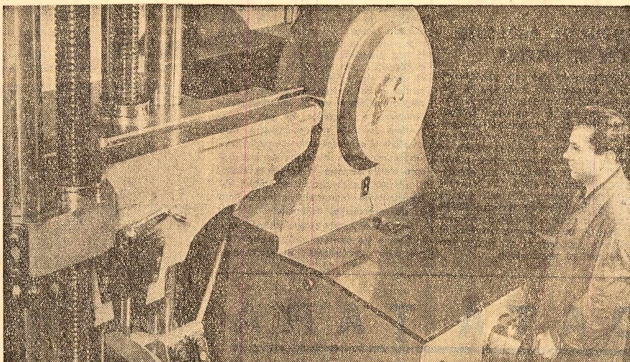
Laboratorul uzinelor „23 August” din Capitală. În vederea înlocuirii avantajose a unor oțeluri aliate cu altele mai ieftine, aici se fac numeroase probe și încercări. În fotografie: So încercă la tracțiune o epruvetă dintr-un nou material pentru arborii cotiți.
