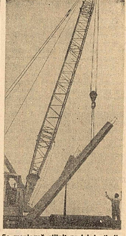
Se montează stîlpi prefabricați din beton armat, turnați pe șantier, la vîntoarea fabricii de befoane celulare autoclavizate.
