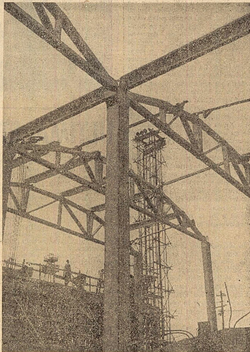
Metodele industriale de construcții sînt tot mai larg extinse pe șantierele Truștului 1 Construcții, în fotografia de față de montaj a stîlpilor și formelor precomprimate la o hală industrială.
