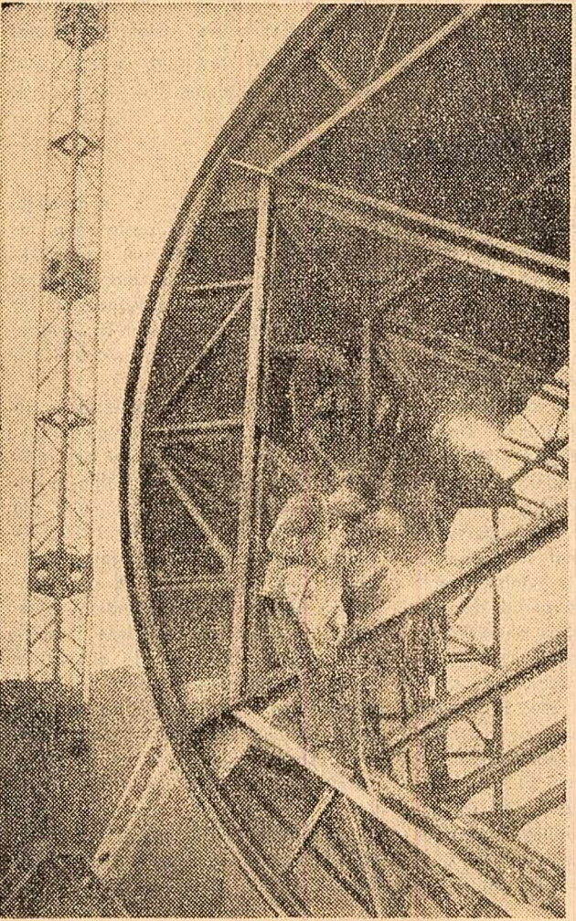
Lucrări de montaj pe șantierul Uzinei de aluminiu Oradea.
