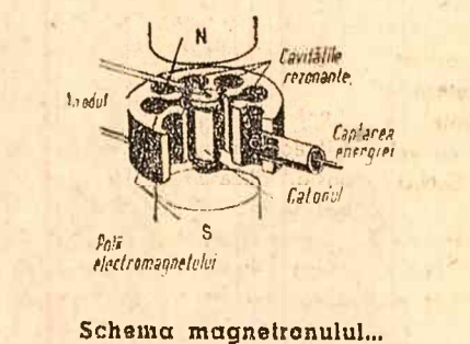
Schema magnetronului...
