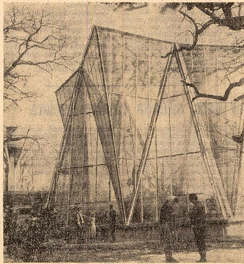
Sera-țur din parcul dendrologic Simeria
