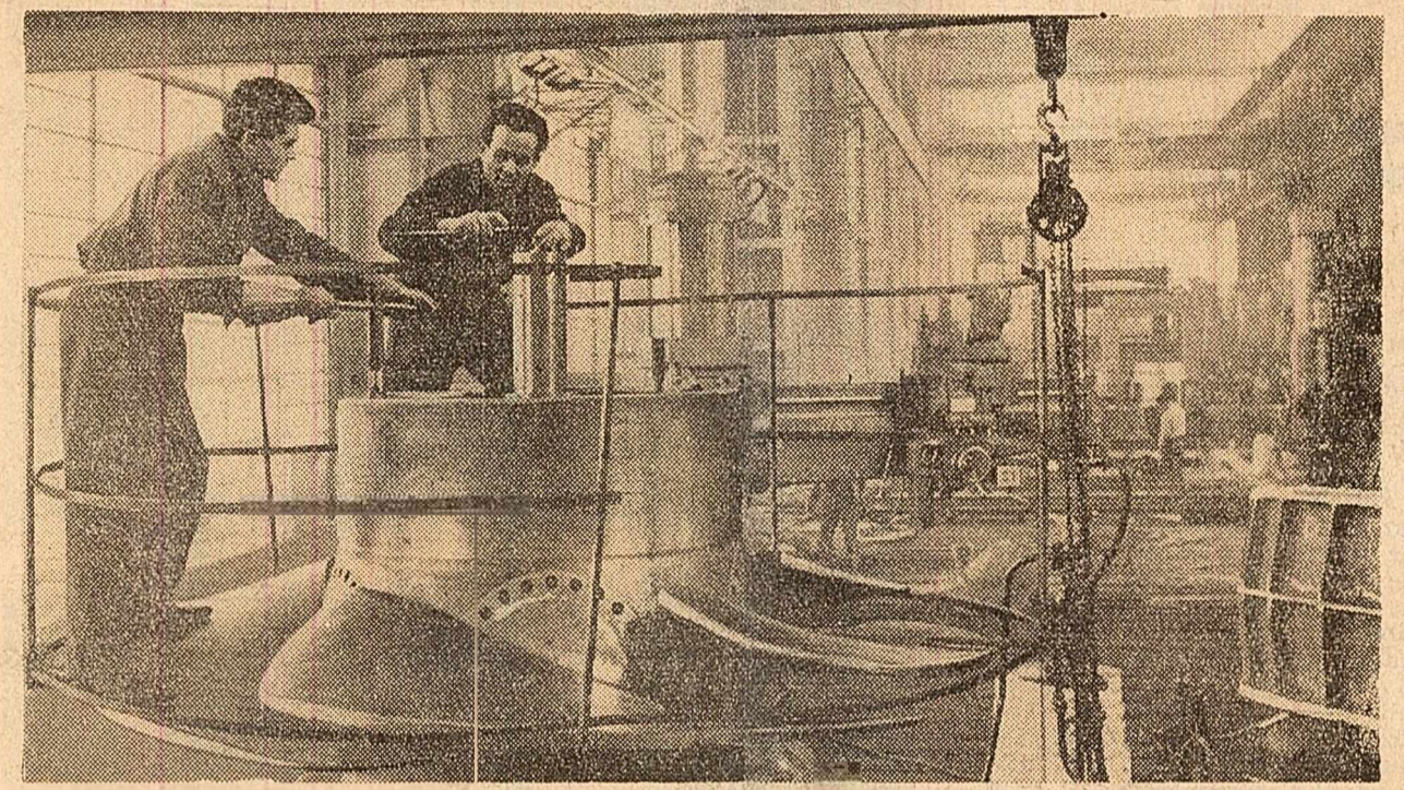
Construcții de mașini de la Reșița desăvârșă o însușeală întrecere pentru îndeplinirea angajamentelor luate în cinstea celei de-a XX-a aniversări a eliberării țării. În centrul întrecerii ei au pus ca un obiectiv principal executarea și livrarea în condiții exemplare a comenzilor pentru marile șantiere. În fotografie: Se lucrează rotorul unei turbine destinate hidrocentralelor ce se construiesc pe Bistrița
